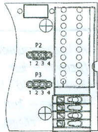
Положение джамперов для тока 100 мА
