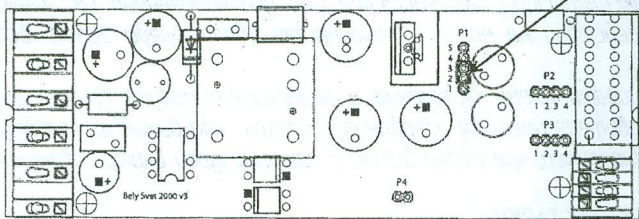
Положение джампера для 1 часа работы в аварийном режиме
