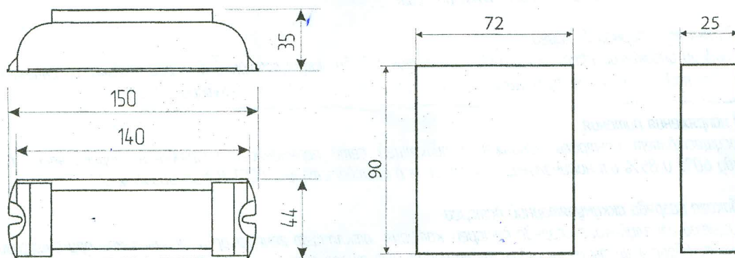
Батарея 6KR23/43-1,5/2F
