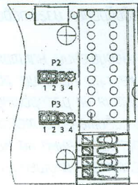
Положение джамперов для тока 150 мА
