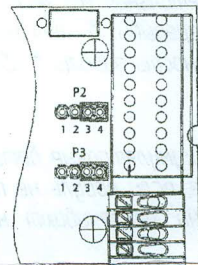
Положение джамперов для тока 350 мА
