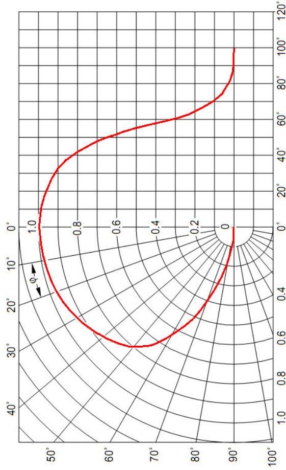
Рисунок 3 Тип КСС в исполнении «Д»
