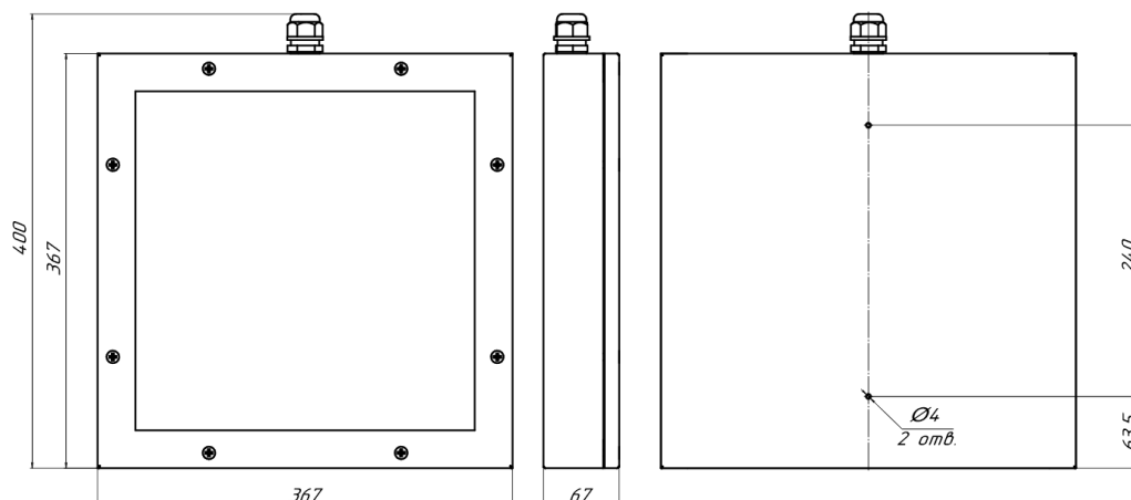
Рис. №2 Габаритный чертёж.
