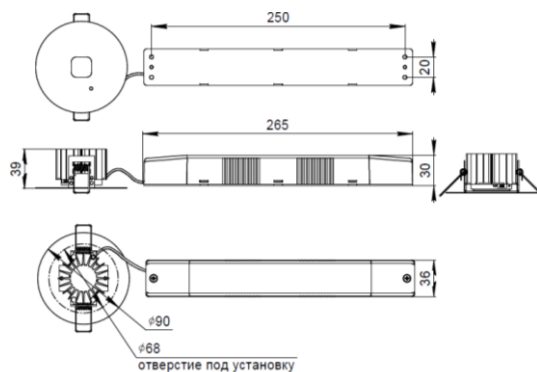
Аварийный светильник BS-ORBITA-81-...
