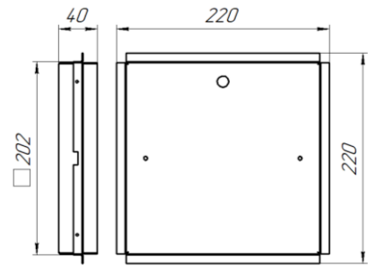
Рис. №3 Бокс стенной BS-BST-7 для заделки в стену
