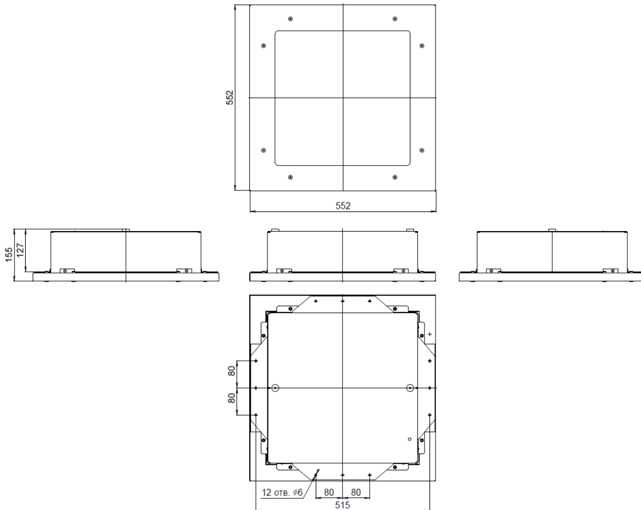
Рис. №5 Габаритный чертёж.
