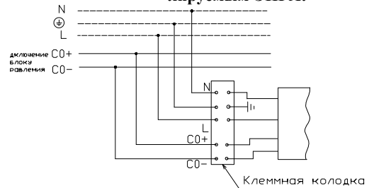
8 Схема подключения к питающей сети с регулируемым ЭПРА:
